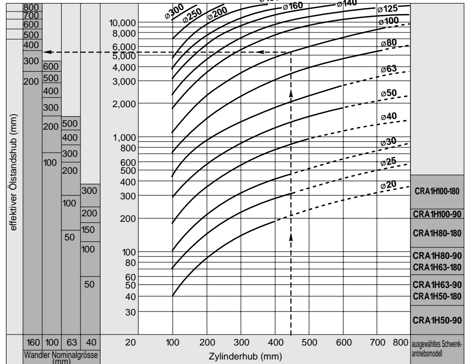
Diagramm A Zylindervolumen/Wandlerkapazität
