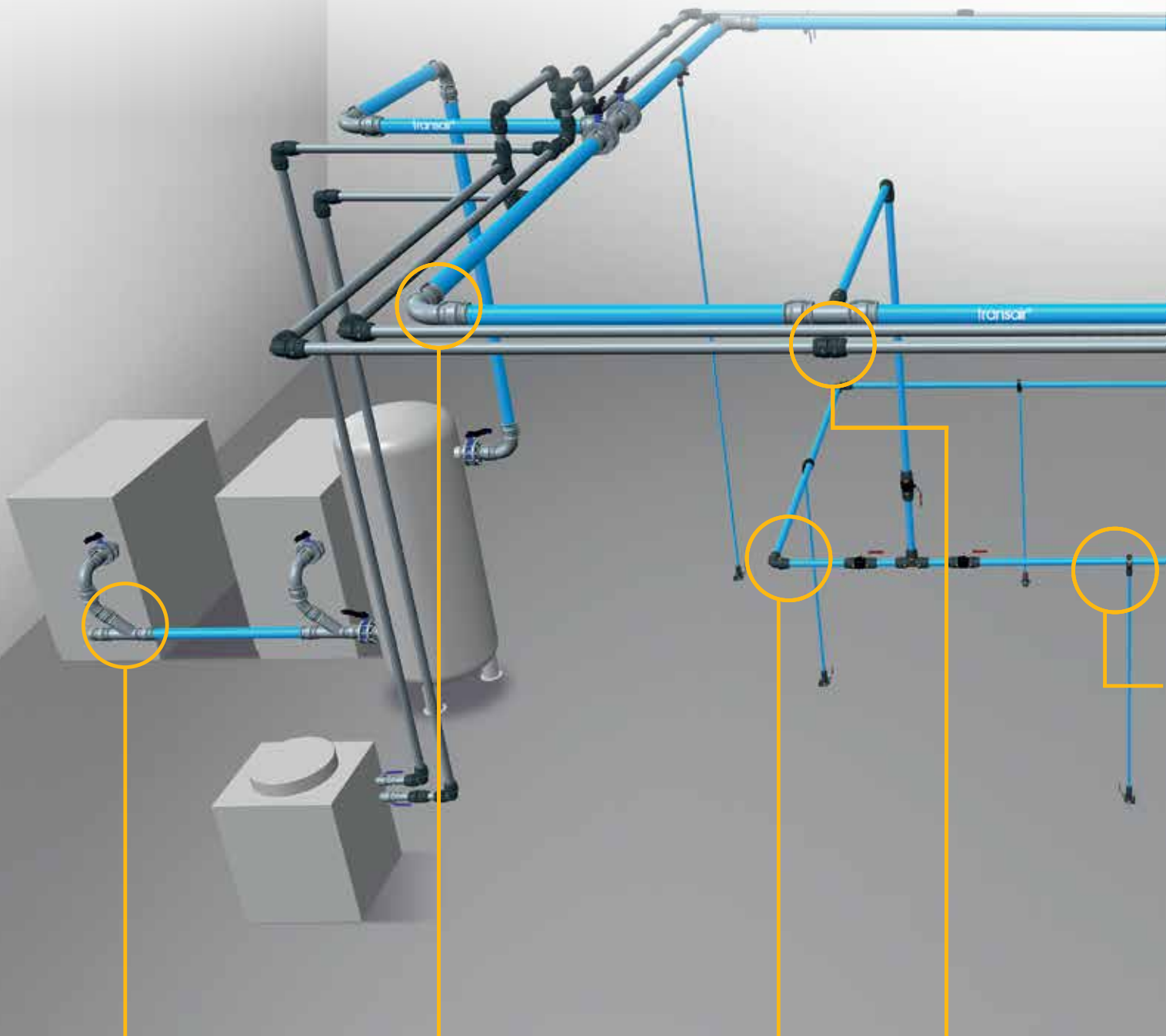
Kompressorraum
