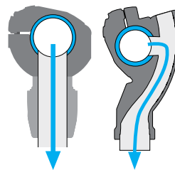
Vertikaler Abgang
