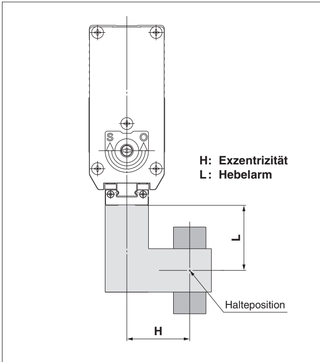
Außengreifend
