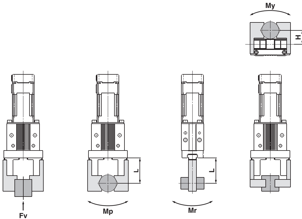
Fv: zulässige vertikale Last Mp: Längsbelastung Mr: Seitenbelastung My: Querbelastung
