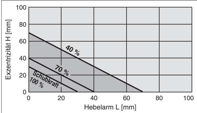
LEHZJ16
