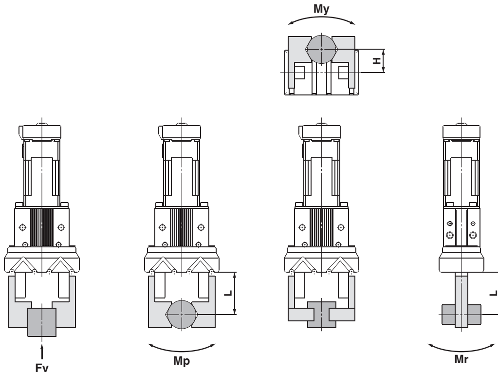
Fv: zulässige vertikale Last Mp: Längsbelastung My: Querbelastung Mr: Seitenbelastung
