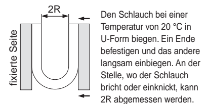
Messung des kleinsten Biegeradius.
