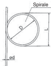
Schlauchverformung bei Anwendung des kleinsten Biegeradius.
